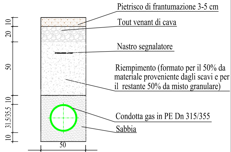
SEZIONE DI SCAVO PER POSA DI CONDOTTA DN 315/355 SU STRADA STERRATA
