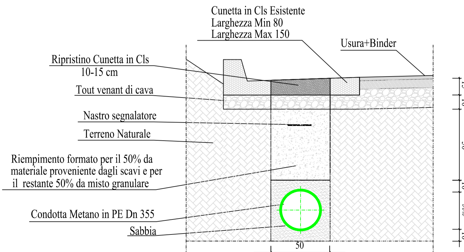
SEZIONE DI SCAVO PER POSA DI CONDOTTA DN 355 SU CORPO STRADALE - ELEMENTO MARGINALE CUNETTA IN CLS
