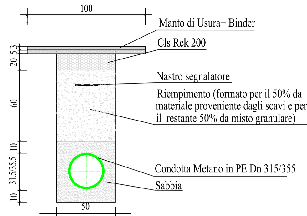
SEZIONE DI SCAVO PER POSA DI CONDOTTA DN 315/355 SU PAVIMENTAZIONE BITUMATA
