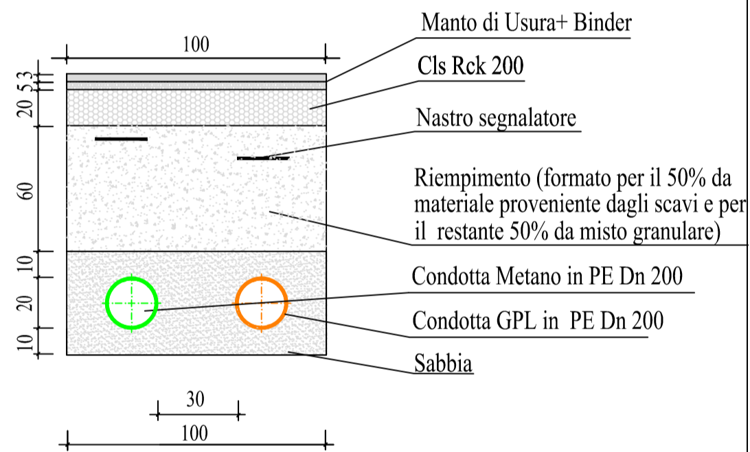
SEZIONE DI SCAVO PER POSA DI CONDOTTA DN 200 SU PAVIMENTAZIONE BITUMATA IN AFFIANCAMENTO A CONDOTTA GPL ESISTENTE
