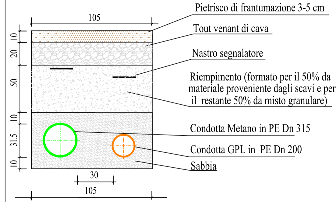
SEZIONE DI SCAVO PER POSA DI CONDOTTA DN 315 SU STRADA STERRATA IN AFFIANCAMENTO A CONDOTTA GPL ESISTENTE
