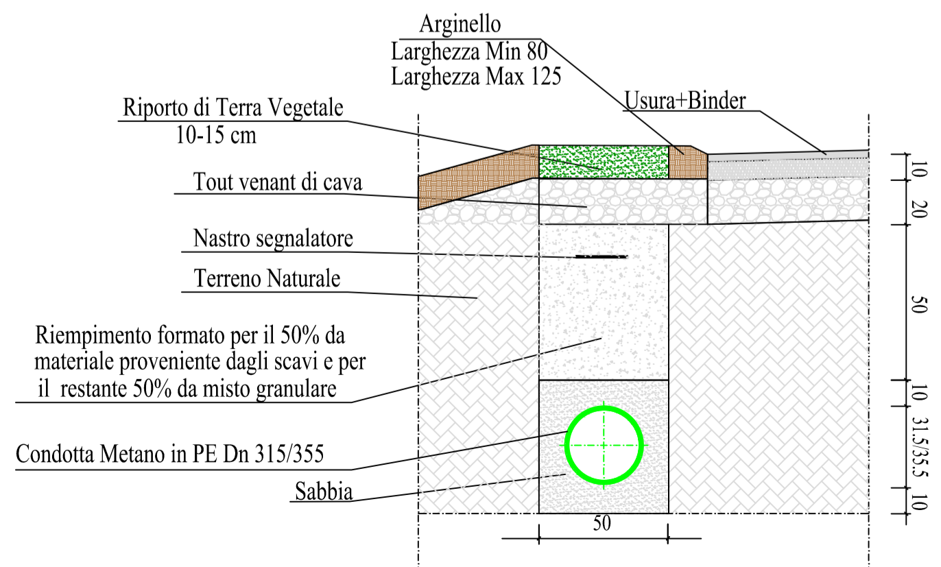
SEZIONE DI SCAVO PER POSA DI CONDOTTA DN 315/355 SU CORPO STRADALE - ELEMENTO MARGINALE ARGINELLO O CUNETTA IN TERRA
