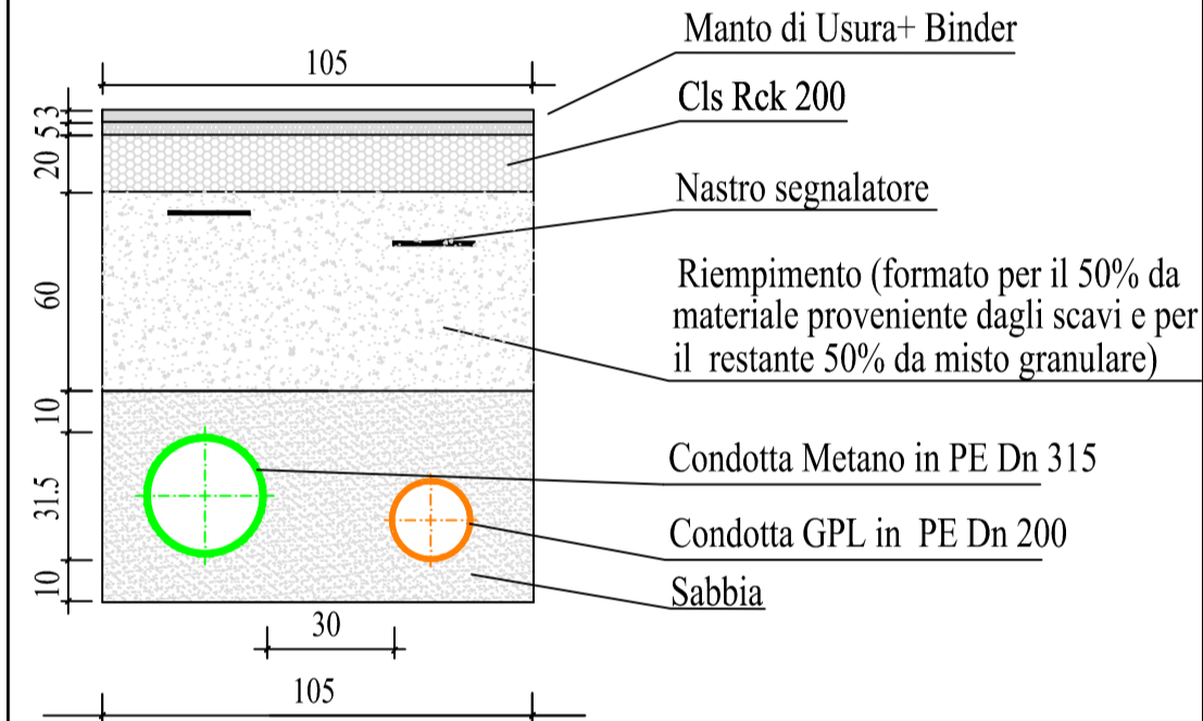
SEZIONE DI SCAVO PER POSA DI CONDOTTA DN 315 SU PAVIMENTAZIONE BITUMATA IN AFFIANCAMENTO A CONDOTTA GPL ESISTENTE
