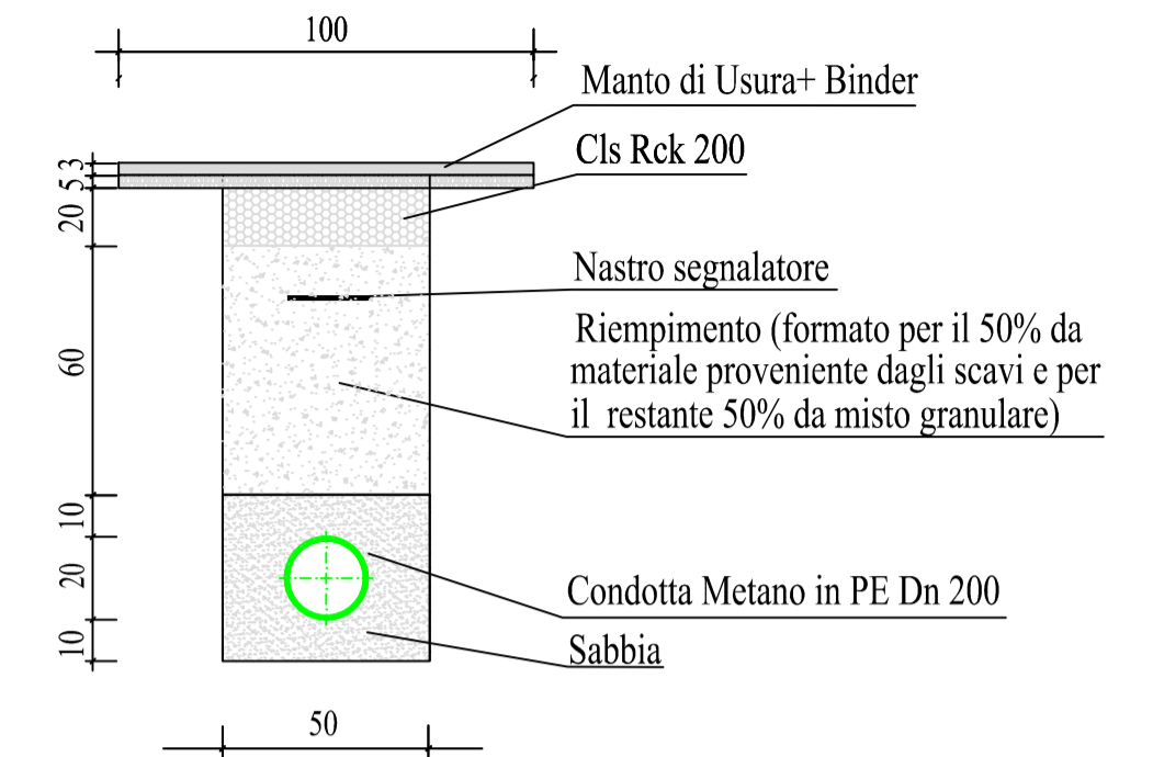
SEZIONE DI SCAVO PER POSA DI CONDOTTA DN 200 SU PAVIMENTAZIONE BITUMATA
